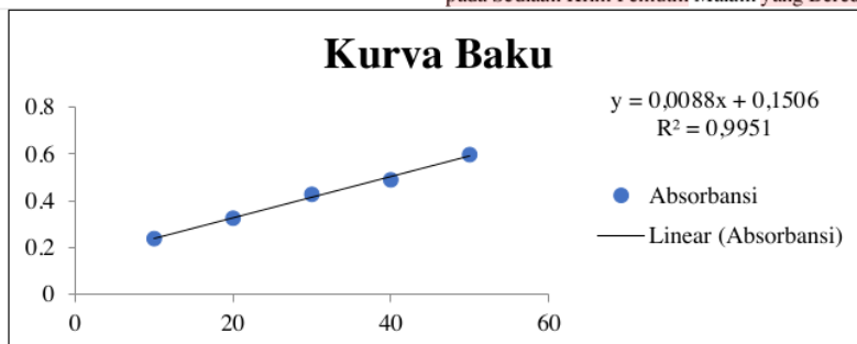
Gambar 3. Kurva Baku
