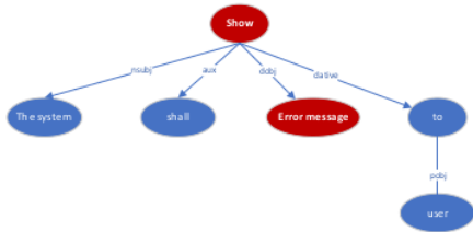
Gambar 5. Pola Kalimat untuk Aturan 1.
