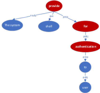
Gambar 6. Pola Kalimat untuk Aturan 2.
