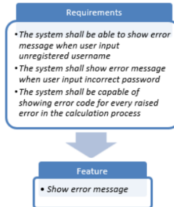
Gambar 3. Ilustrasi Identifikasi Fitur dari Kalimat Pernyataan Kebutuhan (Haris, Kumiawan and Ramdani, 2020)
