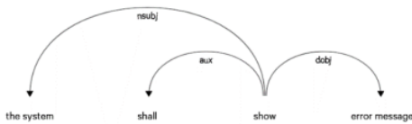
Gambar 2. Ilustrasi Dependency Parser pada NLP menggunakan Spacy
