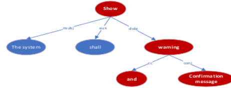
Gambar 7. Pola Kalimat untuk Aturan 3.
