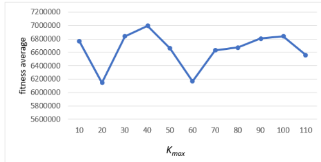
Fig. 8. K_{max} Testing
