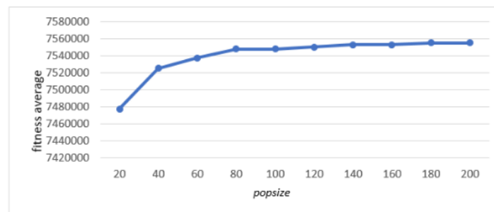
Fig. 5. Popsiz
