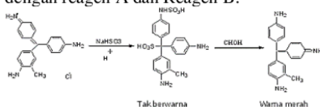
Gambar 3. Reaksi Perubahan Warna antara Formalin dengan Schiff
