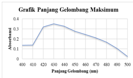
Gambar 1. Grafik panjang gelombang maksimum formalin
