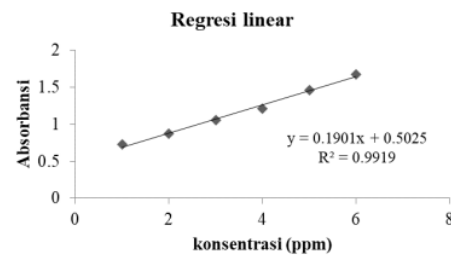
Gambar 2. Kurva Kalibrasi Formalin
