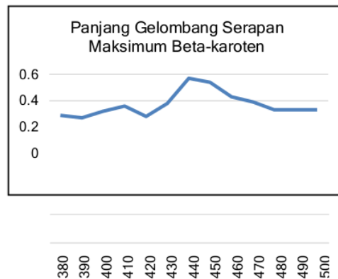
Gambar 1. Panjang gelombang serapan maksimum Beta-karoten standart
